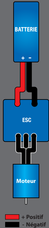
Diagramme de câblage du contrôleur BL-2s
